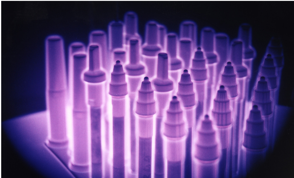
Druckgusskerne während einer Plasmanitrierung. © Fraunhofer IST
